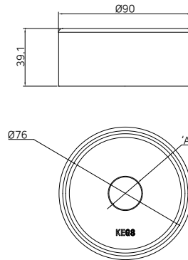
KEG8 시리즈
