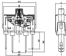
FCB / 접점 블록 (1N/O + 1N/C)
