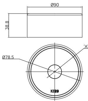
KEG9 시리즈
