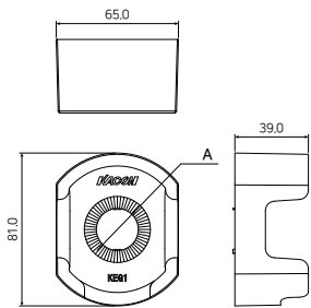
KEG12 / 15 / 13
