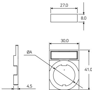
HP110A / HP110B
