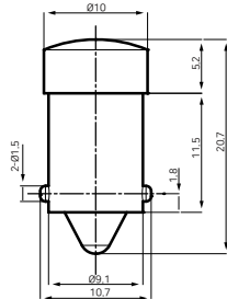
BA9S-J
