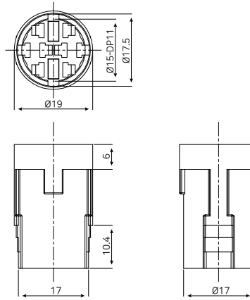
T19 커넥터
