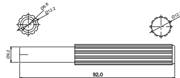
K16 - LR1
