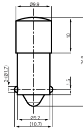
BA9S-K
