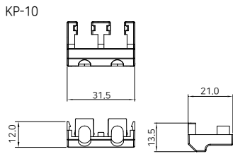
CBA, CBB용 접점안전커버
