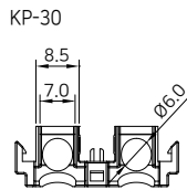
CBA2 CBB2 CBC용 접점안전커버
