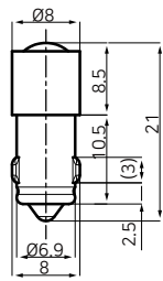
BA7S-K
