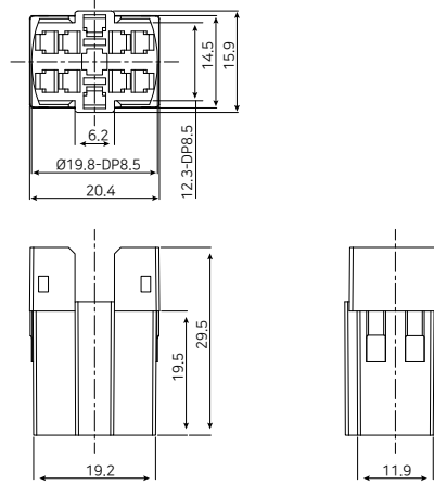
T25 커넥터
