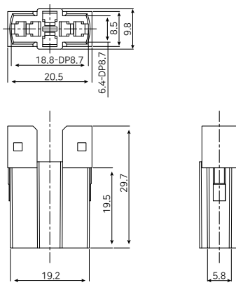
T22 커넥터
