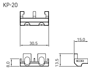
트랜스안전커버
