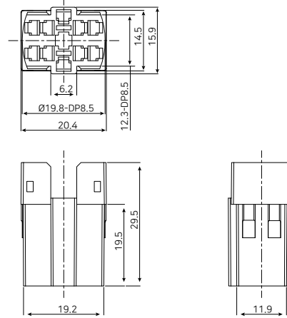
T25 커넥터
