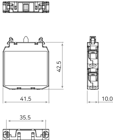
트랜스안전커버
