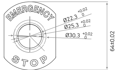
HP119E / HP119K / HP119C / HP119E-R
