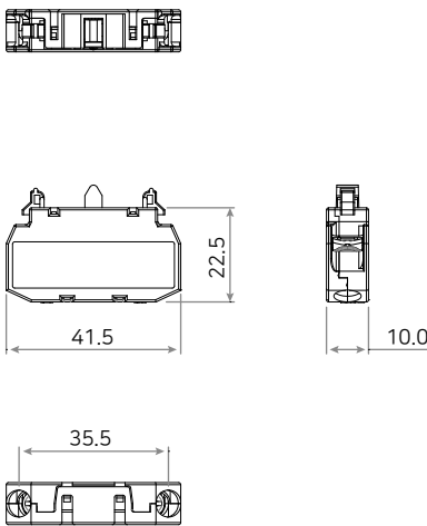
CBA, CBB용 접점안전커버
