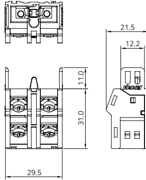
J2-20 / J2-02 / J2-11
