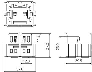
KAL / 자기유지 Holder
