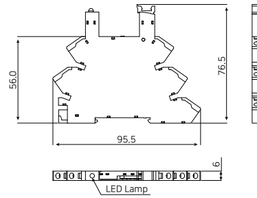
RXT - Q01 핀 타입
