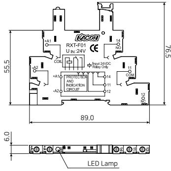
RXT - F01 스크류 타입
